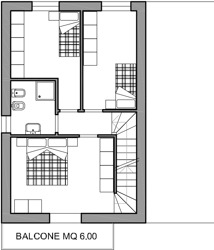
PIANO PRIMO MQ 63
